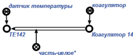
Рисунок 15 - Семантическое представление связи единицы оборудования с его конструктивной частью
