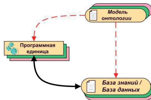
Рисунок 1 – Онтологический двухуровневый подход к формированию данных и знаний: отделение предметных знаний от знаний о методах решения задач
